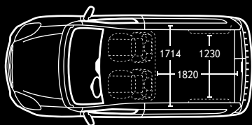
Van z krótkim rozstawem osi i niskim lub wysokim dachem.
