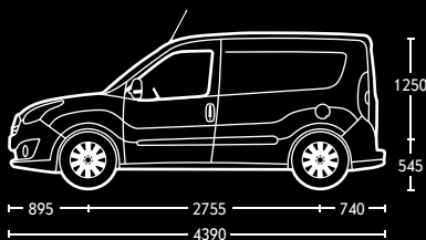
Van z krótkim rozstawem osi i niskim dachem.
