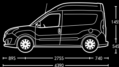
Van z krótkim rozstawem osi i wysokim dachem.
